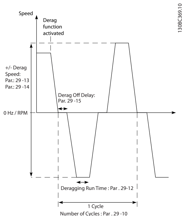
Bild 3.80 Rensningsfunktion
