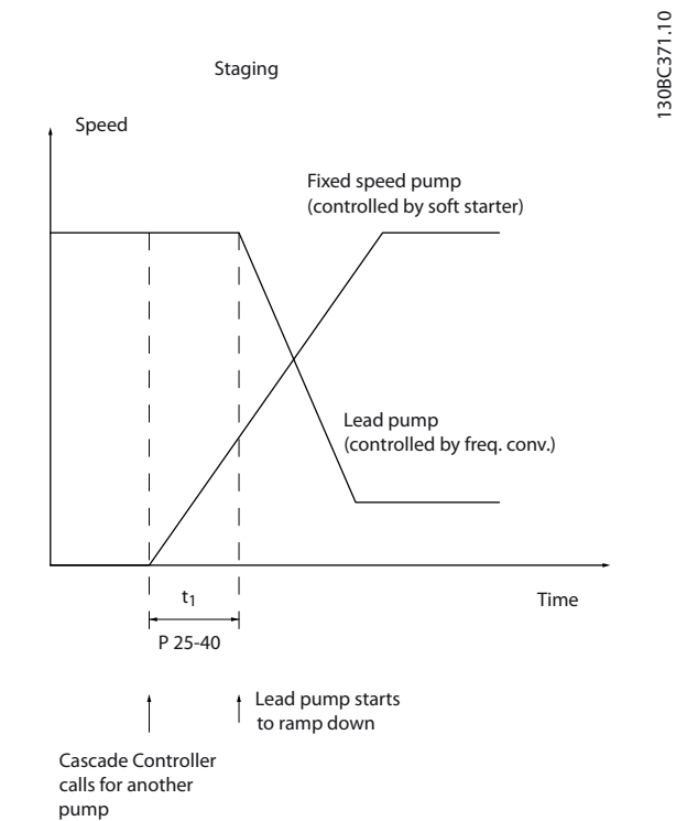
Bild 3.71 Inkoppling
