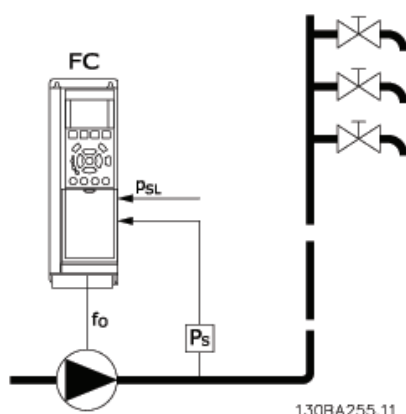
Bild 3.48 Skala: FC = frekvensomformare, f_0 =utfrekvens, P_S =P-system, P_{SL} =P-börvärde
