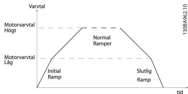
Bild 3.15 Inledande och avslutande ramptid
