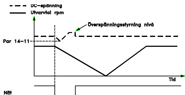
Bild 3.34 Kontrollerad nedrampn - Kort nätfel. Nedrampn till stopp följt av upprampning till referens.
