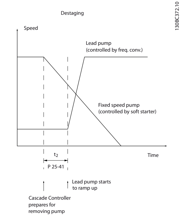
Bild 3.72 Urkoppling
