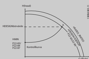
Bild 3.54 Varvtal vid systemdesignsarbetsgränsen är känd
